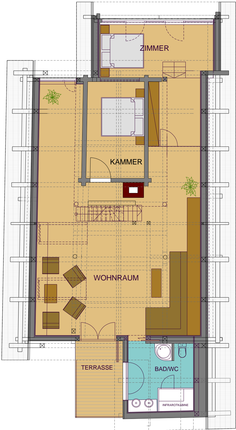
1. OBERGESCHOSS
